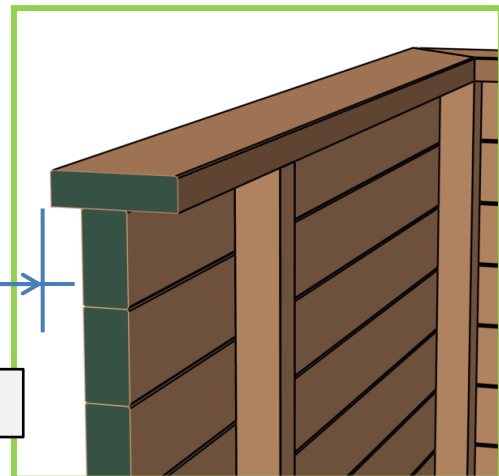
Querschnitt durch den Handlauf
